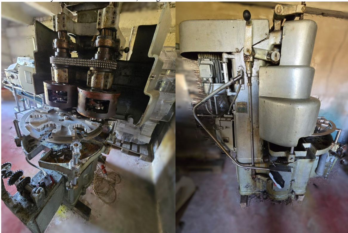
14. Закочувальна машина Тріо Норвегія з клінчером, налаштована на алюмінієву банку клуб. 14. Trio Norway can seamer with clincher, configured for aluminum club cans.
